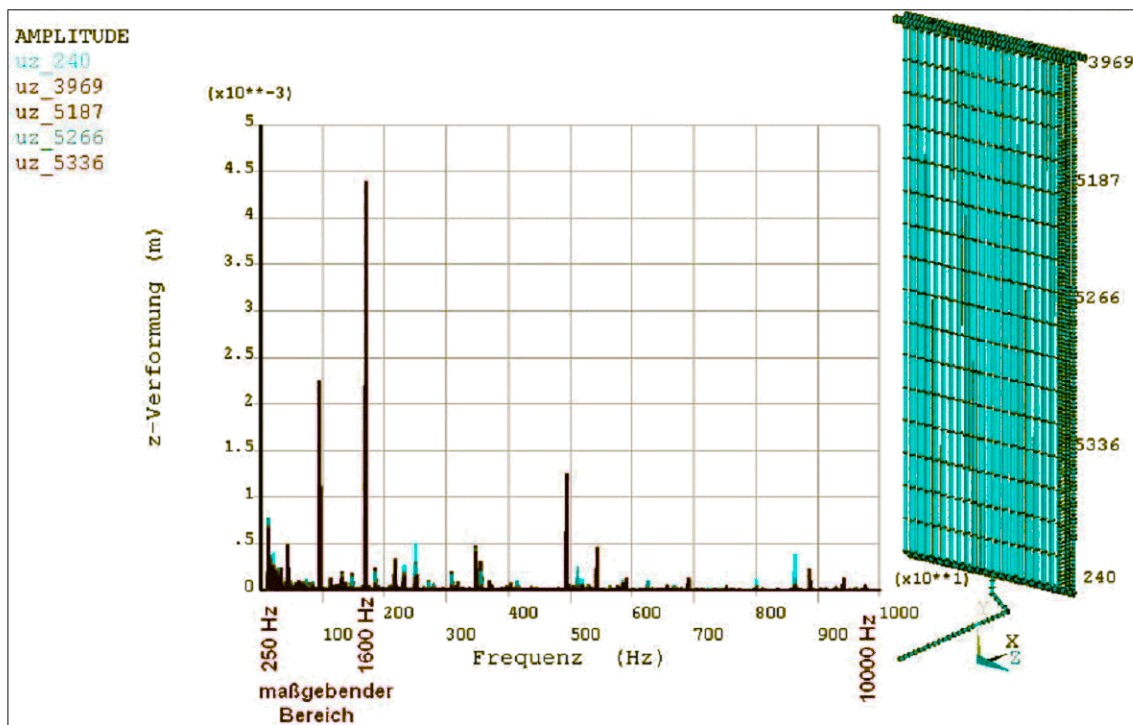
Abb. 15: Frequenzganganalyse
