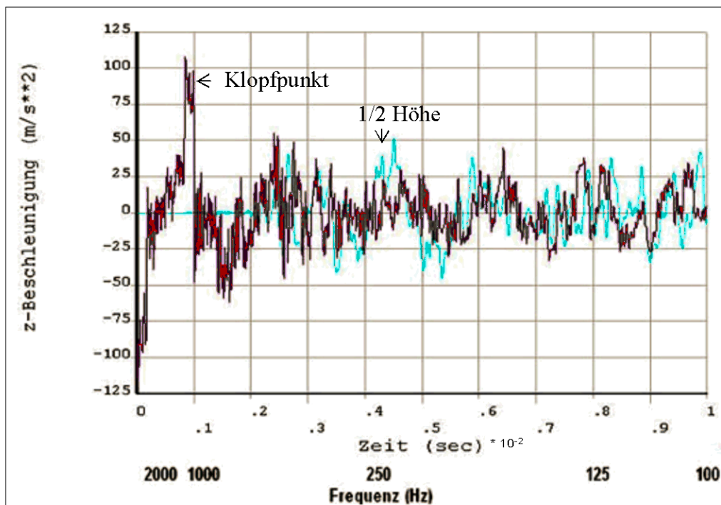
Abb. 14: Beschleunigung der Harfe am Klopfpunkt (unten) und auf halber Höhe.
