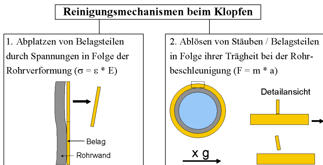
Abb. 12: Wirkmechanismen der Klopfung (links: Verformung, rechts: Trägheit)
