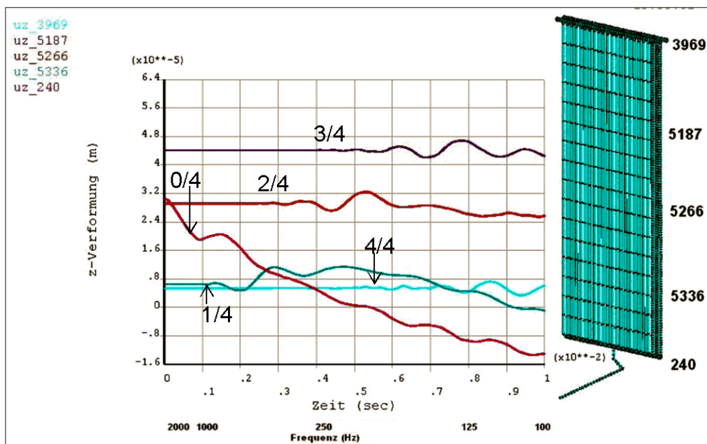
Abb. 13: Verformung der Harfe in verschiedenen Höhen (0/4 = unten; 4/4 = oben)
