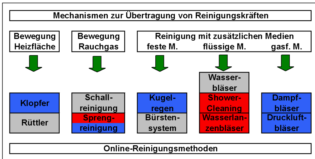
Abb. 2: Online-Reinigungsmethoden gegliedert nach dem Medium zur Kraftübertragung
