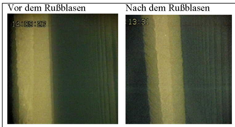
Abb. 10: Anströmseite eines Überhitzerbündels
