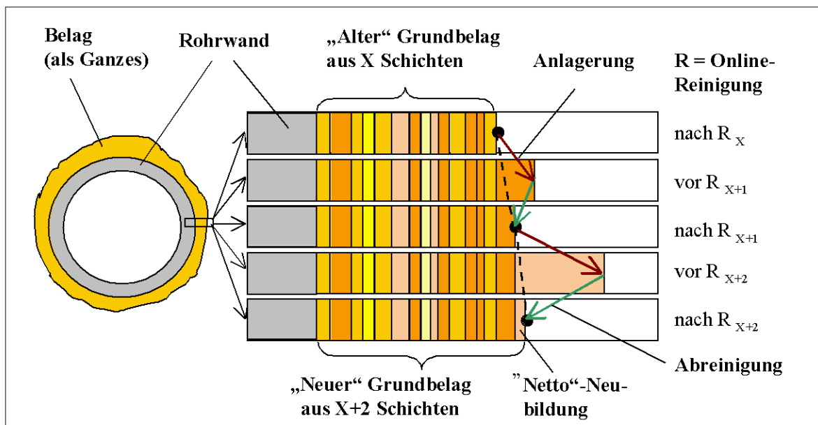
Abb. 19: Schema „Quasikontinuierliche Belagsbildung“
