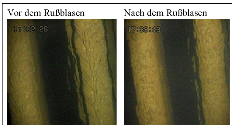
Abb. 11: Anströmseite einer Verdampferfahne
